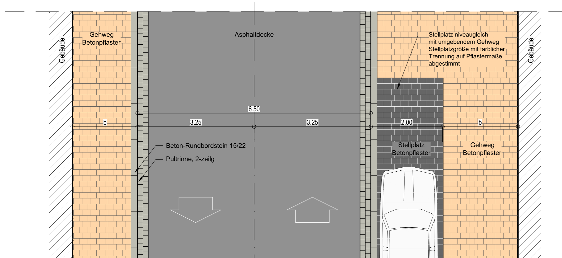
Lageplanauszug M. 1:50
